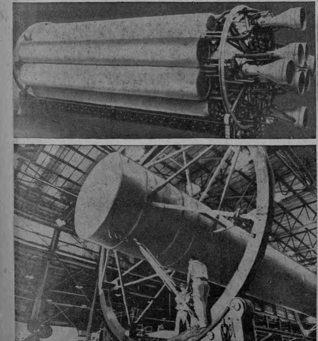
VEHICULO DEL ESPACIO.—Arriba aparece la escala de un cuarto de la primera etapa del gigante vehículo del espacio "Saturno", en Huntsville, Alabama. Abajo, los obreros continúan la fabricación de la sección central de 105 pulgadas. Una vez que esté terminado el "Saturno" se espera que alcance 200 pies de altura y que pese 580 toneladas. El vehículo no será enviado al espacio por lo menos hasta 1963 y será lanzado desde Cabo Cañaveral, en Florida.
